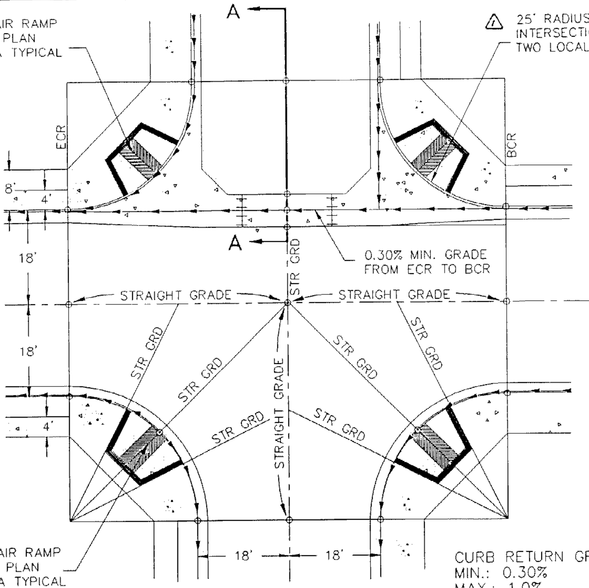
PLAN N.T.S.
